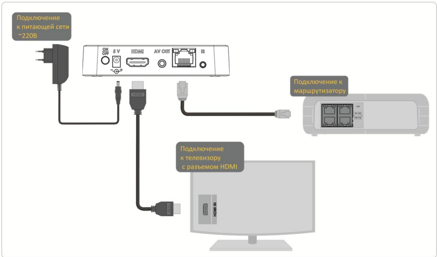
Рисунок 12 — Пример подключения медиацентра
