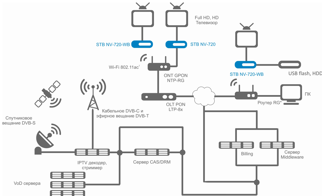
Рисунок 1 — Схема применения
