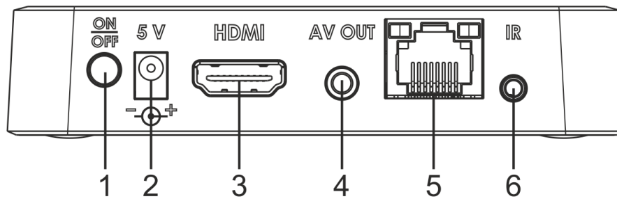
Рисунок 3 – Внешний вид задней панели устройства
