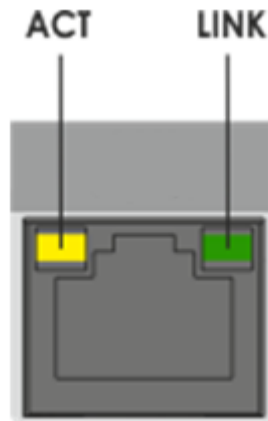
Рисунок 4 — Внешний вид разъема RJ-45
